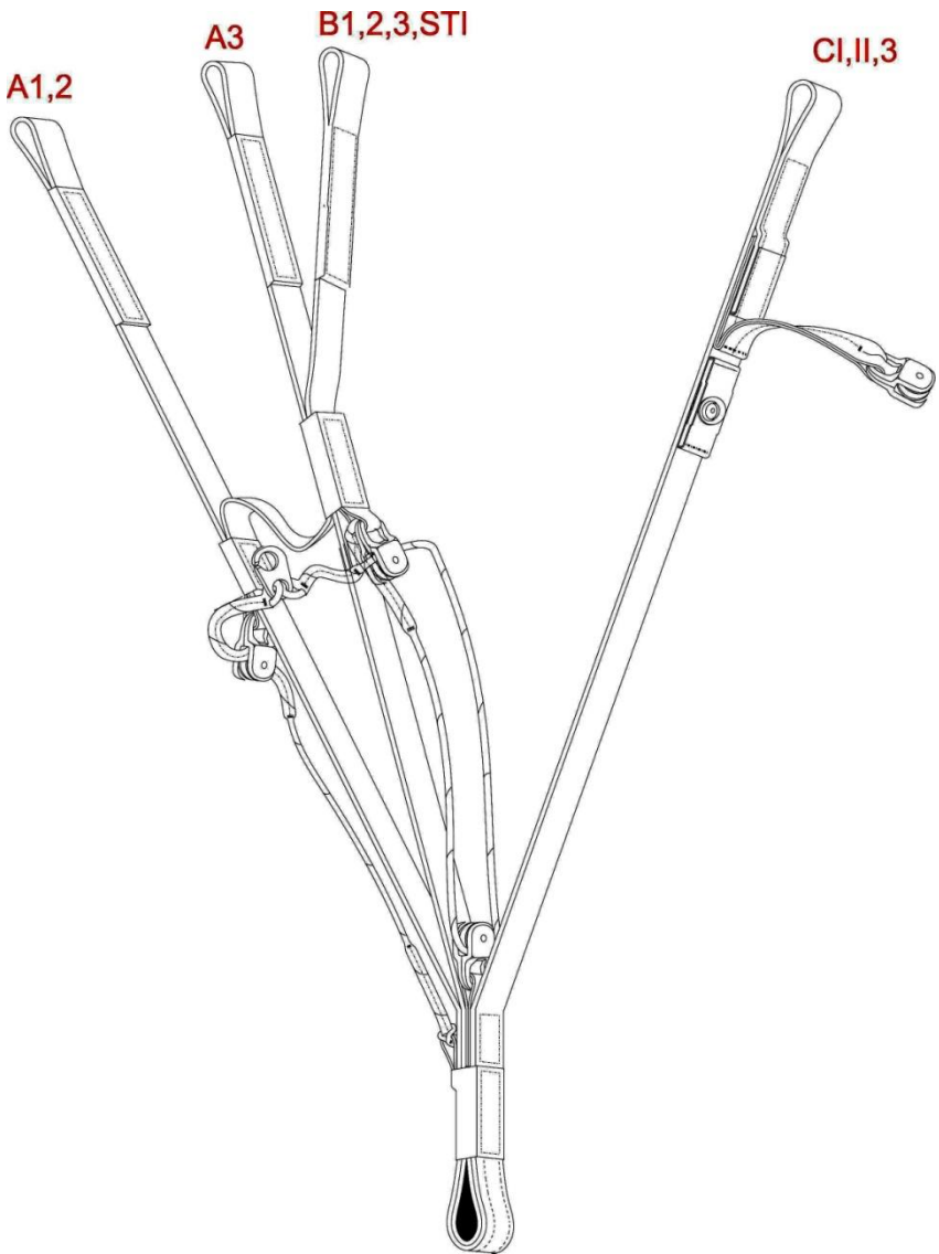
Abbildung 2: Tragegurte des UP Summit XC 2
